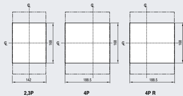
Corte frontal del panel
