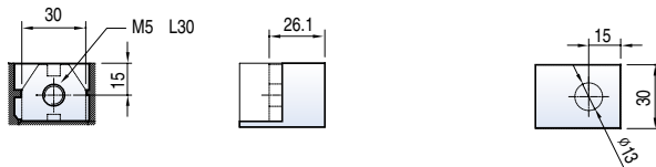
Seccion del terminal
